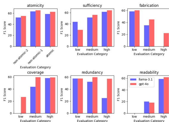
Hình 2: Tác động của các chỉ số chất lượng phụ-tuyên đến hiệu suất xác minh. Xem Phụ lục E để biết chi tiết.
