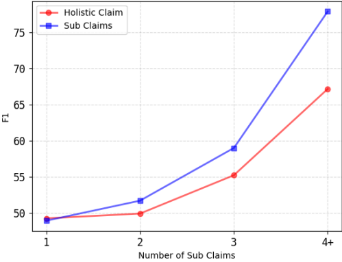
Hình 3: Khi độ phức tạp (tức là số lượng các tuyên bố phụ) tăng lên, hiệu suất của việc phân tích các tuyên bố phụ cải thiện đáng kể.
