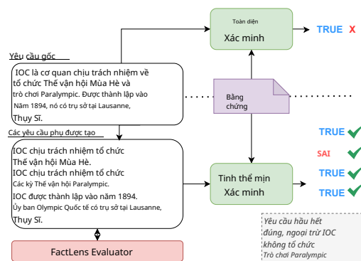
Hình 1: Các ví dụ về xác minh sự thật toàn diện (phía trên) không phát hiện được các sai sót, trong khi xác minh chi tiết (phía dưới) rõ ràng chỉ ra các nguồn lỗi. Trong xác minh chi tiết, Bộ đánh giá FactLens có thể được sử dụng để đánh giá từng tuyên bố phụ và xác định bất kỳ tín hiệu cảnh báo nào có thể gợi ý sự cần thiết phải can thiệp của con người hoặc tái tạo các tuyên bố phụ.
